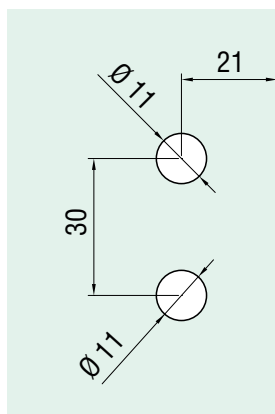
SCHÉMA DE PERÇAGE BORD BOORSHEMA VITRINEWAND
