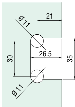
SCHÉMA DE PERÇAGE VANTAIL BOORSHEMA VITRINEDEUR
